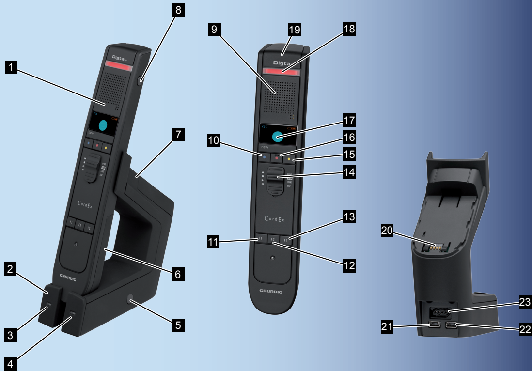
Bild 1: Bedienelemente und Anschlüsse des Diktiermikrofons und der Dockingstation
